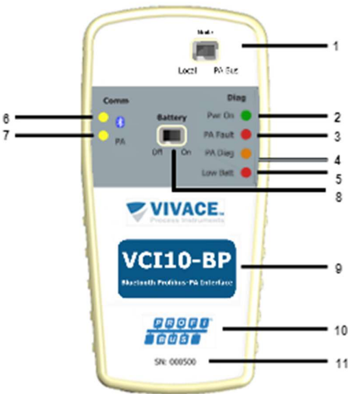
Figura 5.1 – Etiqueta VC110-BP.
